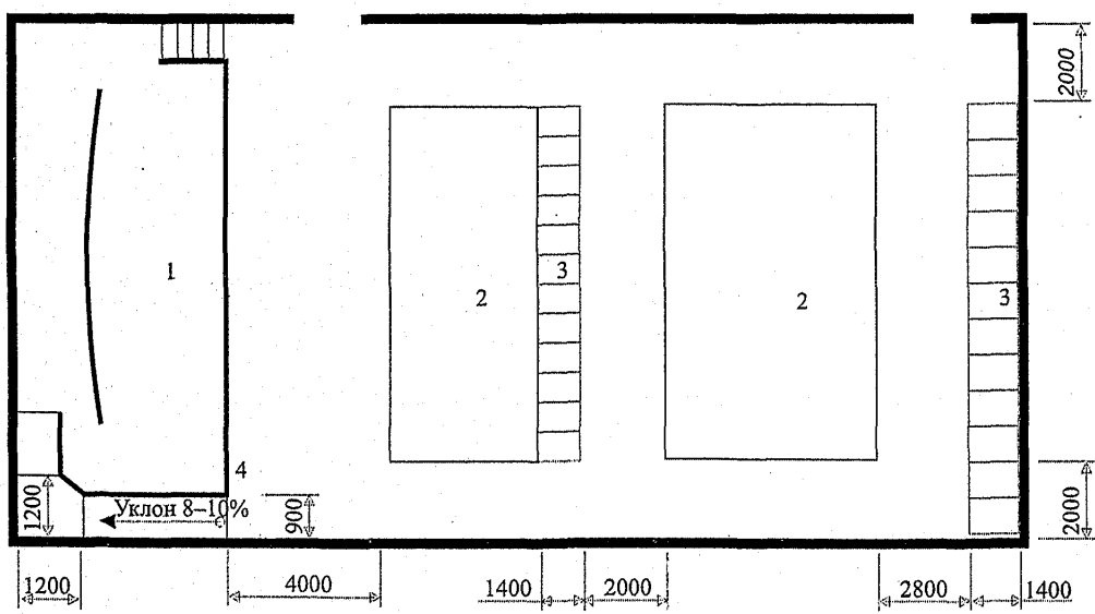
Рисунок Б.10 – Варианты размещения мест в зрительном зале
