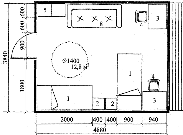
Рисунок Б.5 – Планировочные схемы комнат жилых ячеек ЖЯ-4 для двух- и трехместных комнат
