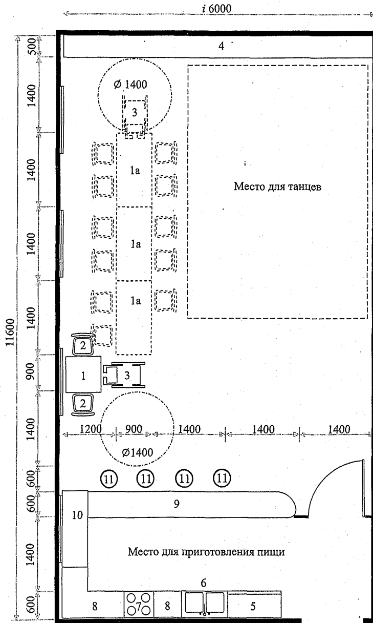
1 – стол обеденный; 1a – стол резервный; 2 – стул; 3 – кресло-коляска; 4 – комбинированная стенка; 5 – холодильник; 6 – мойка; 7 – плита; 8 – буфет кухонный; 9 – сервировочная стойка; 10 – разделочный стол; 11 – табурет
