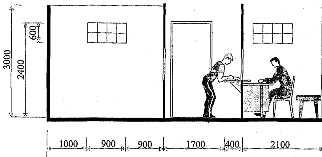
Разрез 1-1
